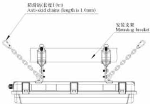
支架式安装 Bracket
