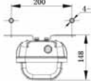
吸顶式安装 II Ceiling type II
