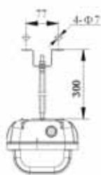
吊杆式安装 Pendant type
