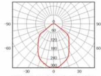
M087D-J70W 金属卤化物灯 Metal halide lamp
