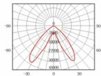
M087D-J1000W 金属卤化物灯 Metal halide lamp
