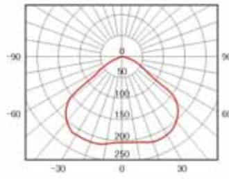
M087D-J250W 金属卤化物灯 Metal halide lamp
