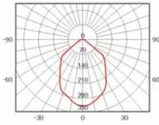
M087D-J150W 金属卤化物灯 Metal halide lamp
