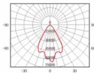
M087D-J1000W 金属卤化物灯 Metal halide lamp
