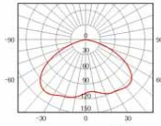
M087D-JN65W 节能灯 Energy-saving lamp
