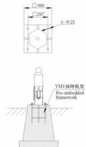
路灯混凝土基础示意图 Street light concrete base diagram
