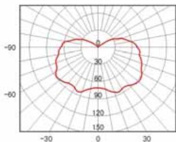
CZ0871-JN45W 节能灯 Energy-saving lamp
