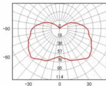
CZ0871-JN65W 节能灯 Energy-saving lamp
