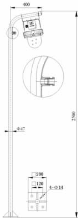
法兰式安装 Flange type
