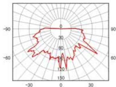
CZ0871-B200W 白炽灯 Incandescent lamp
